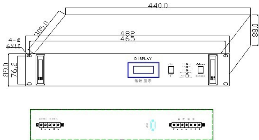
图 1-1 2400 系列 外形示意图
