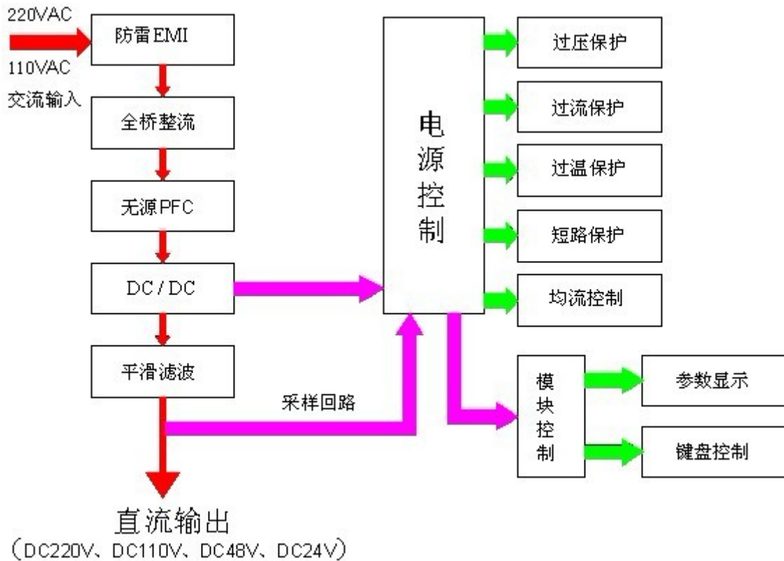
图 2-5 2400 系列原理框图
