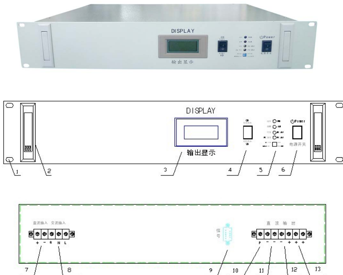
图 2-1 前面板和后面板示意图
