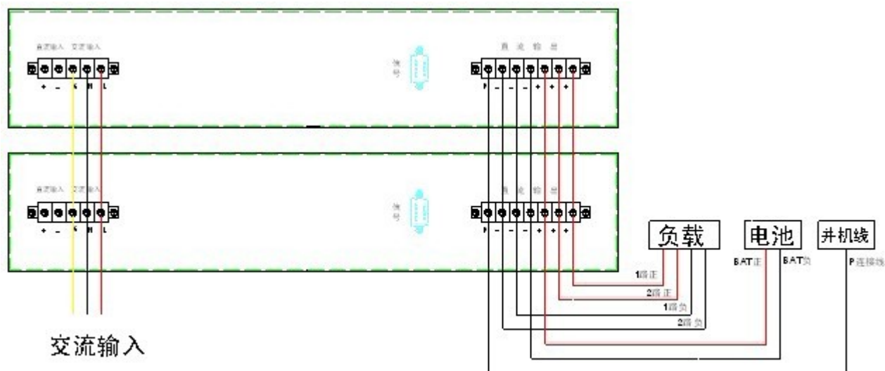
图 3-2 2400 系列高频开关整流器多台并联安装示意图
